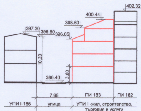
РАЗРЕЗ 4 - 4
