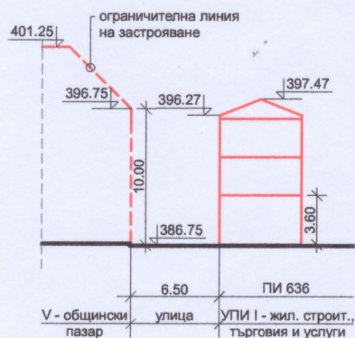
РАЗРЕЗ 6 - 6
