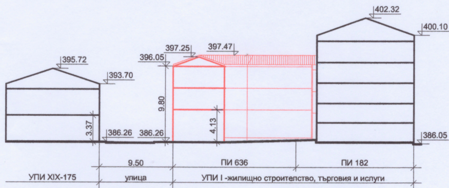
РАЗРЕЗ 5 - 5
