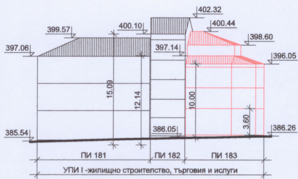
СИЛУЕТ 1 - 1
