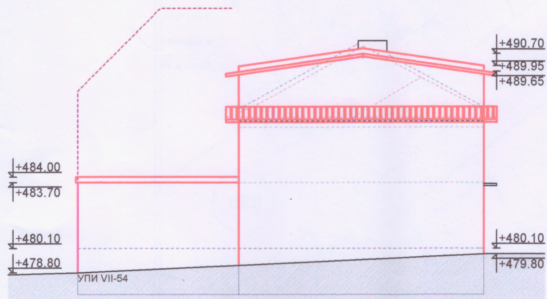
СИЛУЕТ СЕВЕРОЗАПАД ПРЕЗ УПИ VII-54 М 1:200
