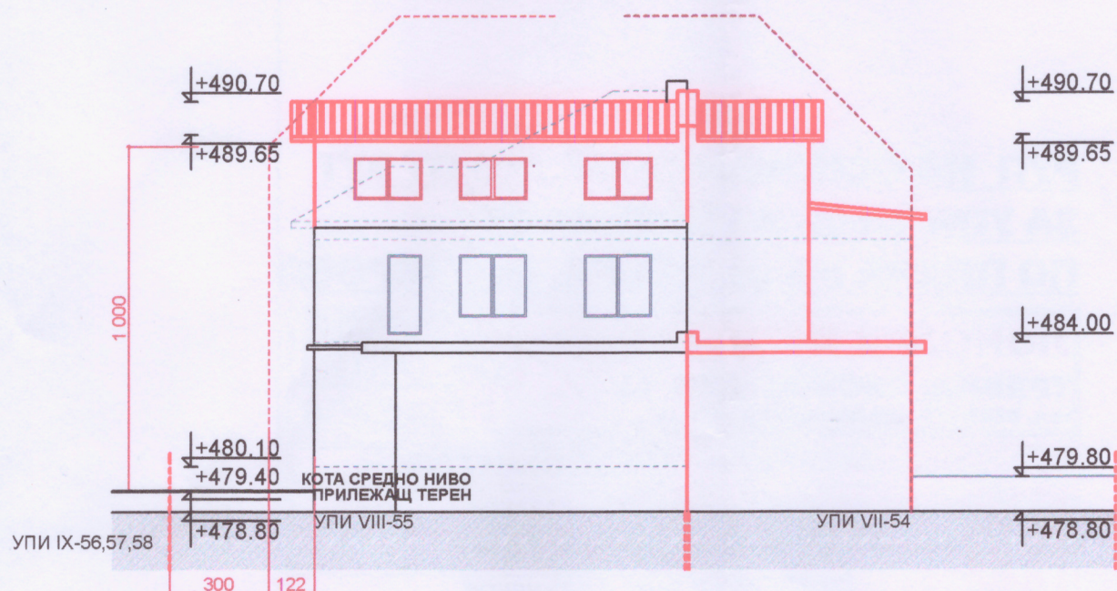
СИЛУЕТ СЕВЕРОИЗТОК ПРЕЗ УПИ VII-54 И VIII-55 М 1:200
