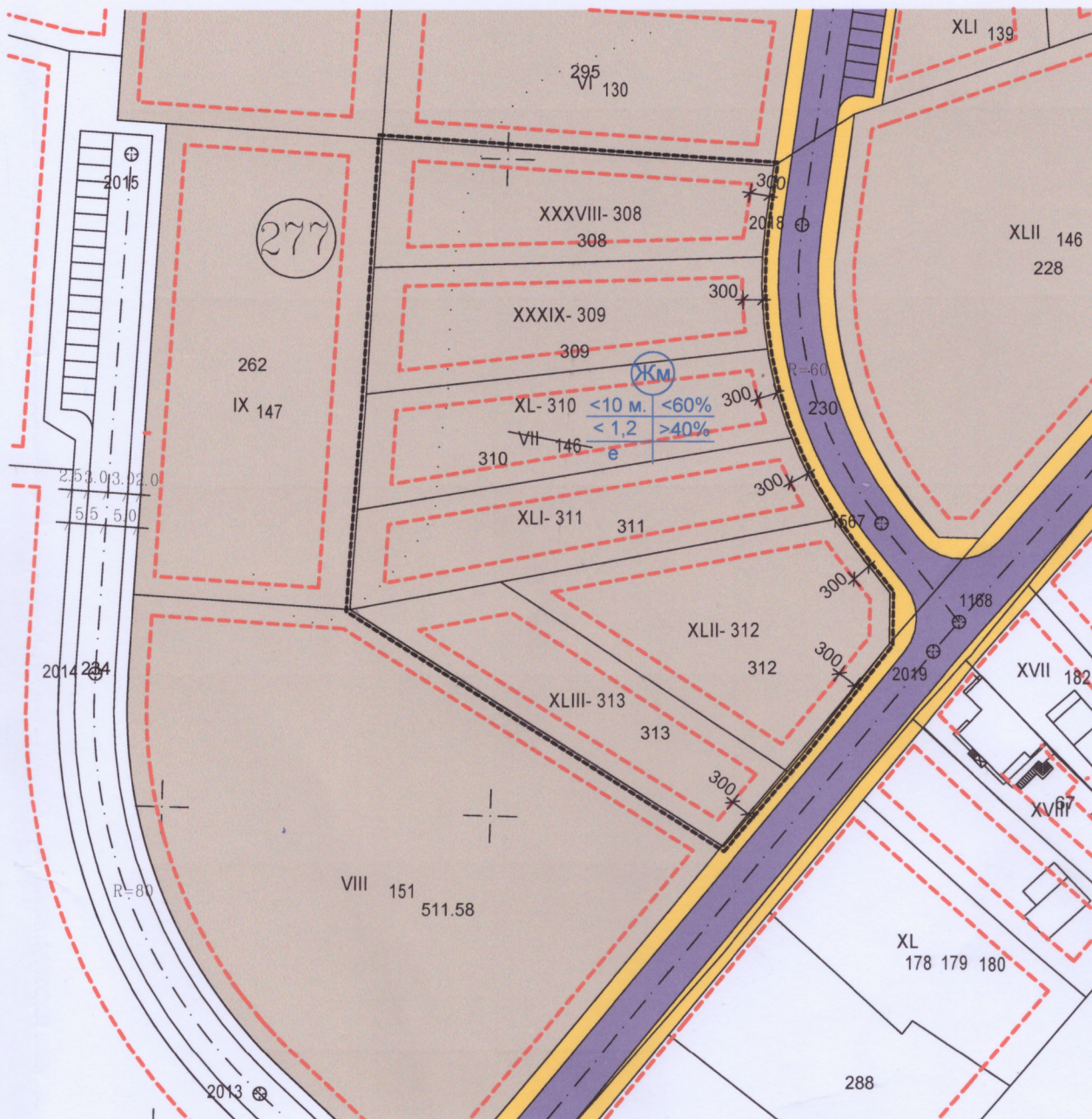
ПОДРОБЕН УСТРОЙСТВЕН ПЛАН- ПЛАН ЗА ЗАСТРОЯВАНЕ М 1: 1000
