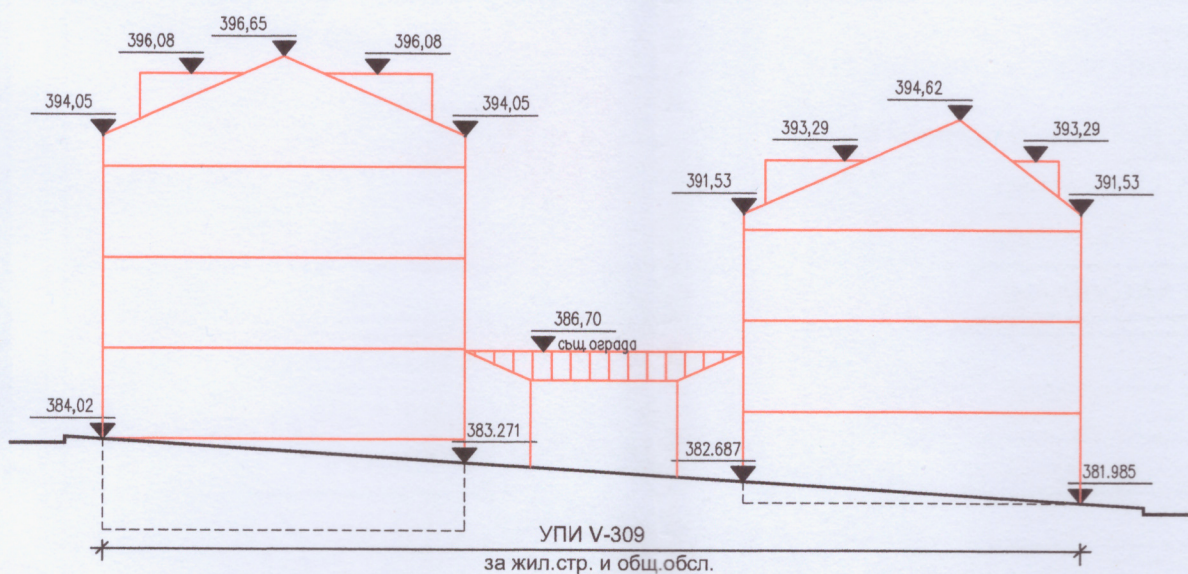
РАЗРЕЗ 1-1 М 1:250
