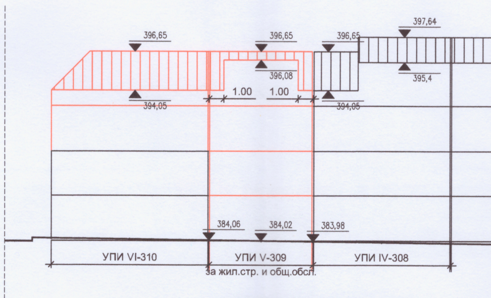
СИЛУЕТ ОТ ИЗТОК М 1:250 ул. "Орловска"
