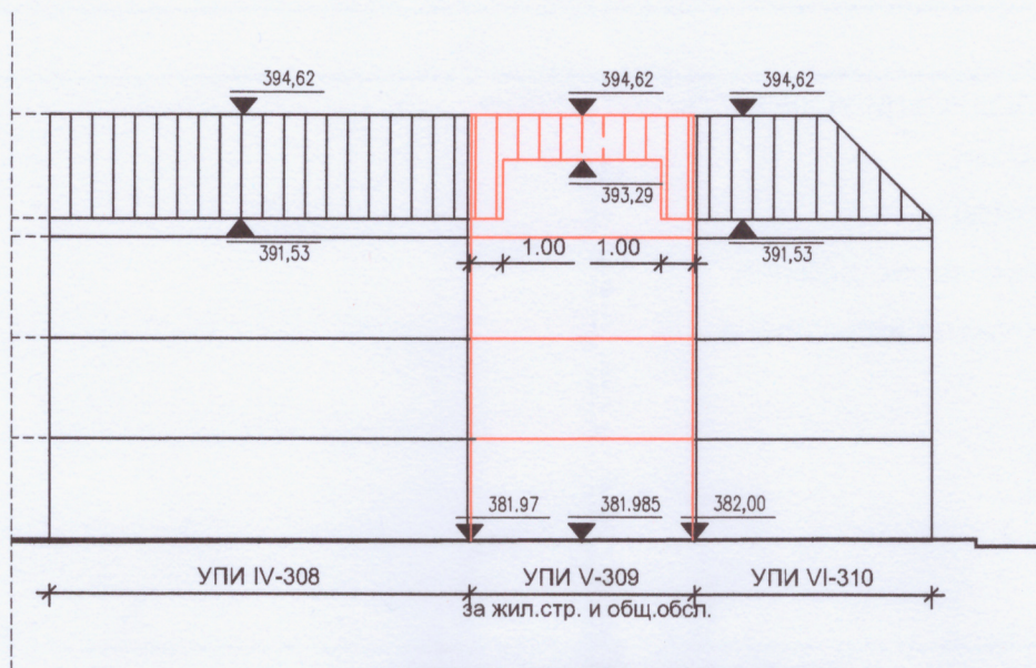
СИЛУЕТ ОТ ЗАПАД М 1:250 ул. "Дунав"
