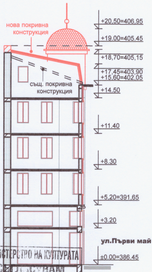
РАЗРЕЗ Б-Б М 1:200
