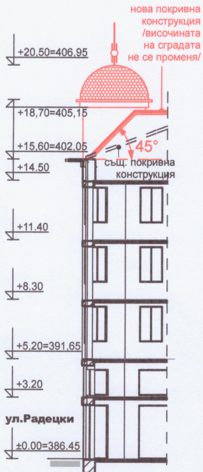
РАЗРЕЗ А-А М 1:200
