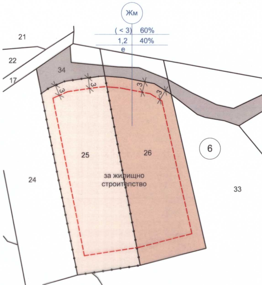
План за застрояване за промяна предназначението на земеделска земя в ПИ 02347.6.25 за разширяване на площадка в ПИ 02347.6.26 по КК на с. Балани М 1:500
